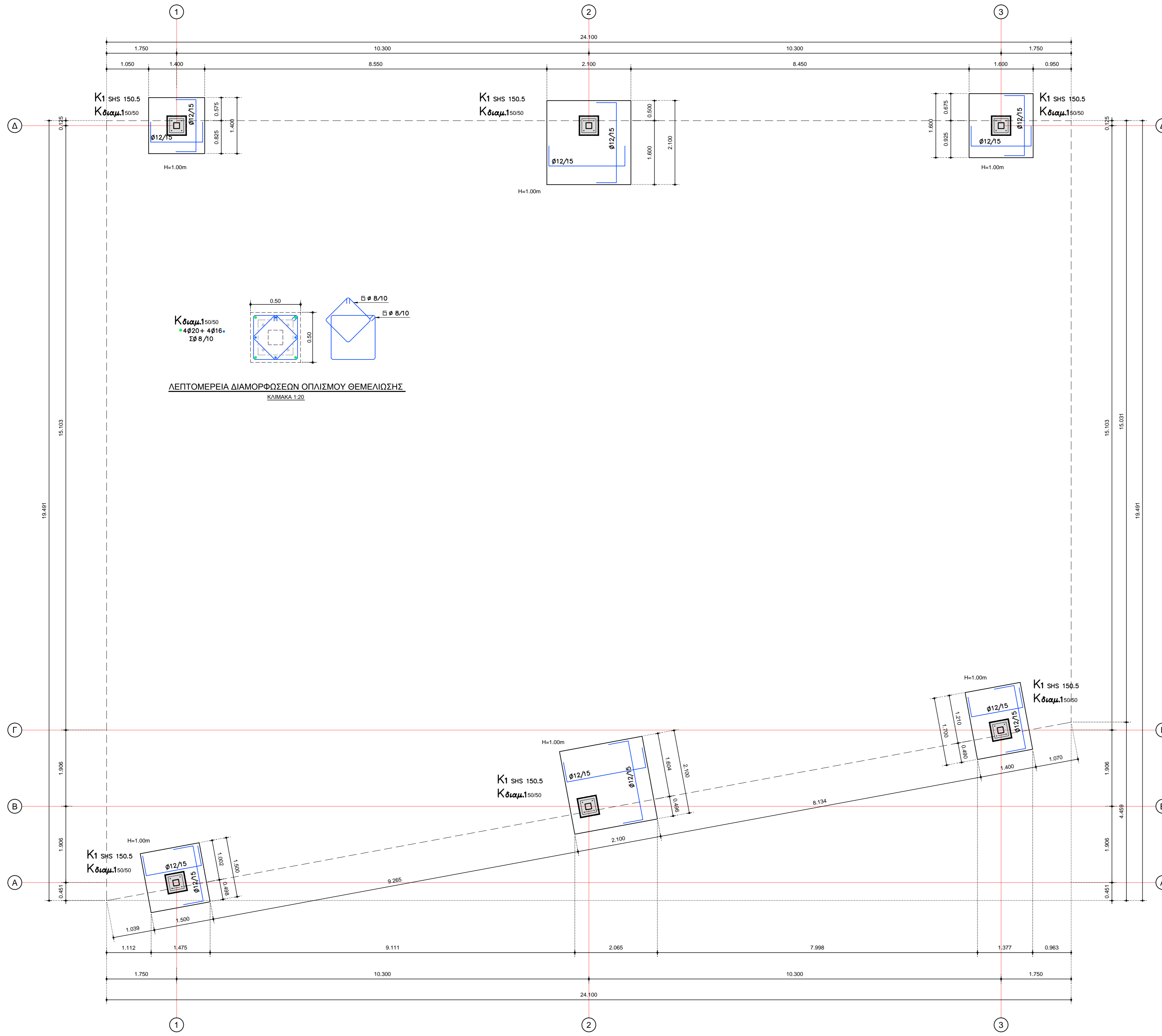
ΘΕΜΕΛΙΩΣΗ ΚΑΙΜΑΚΑ 1:50
