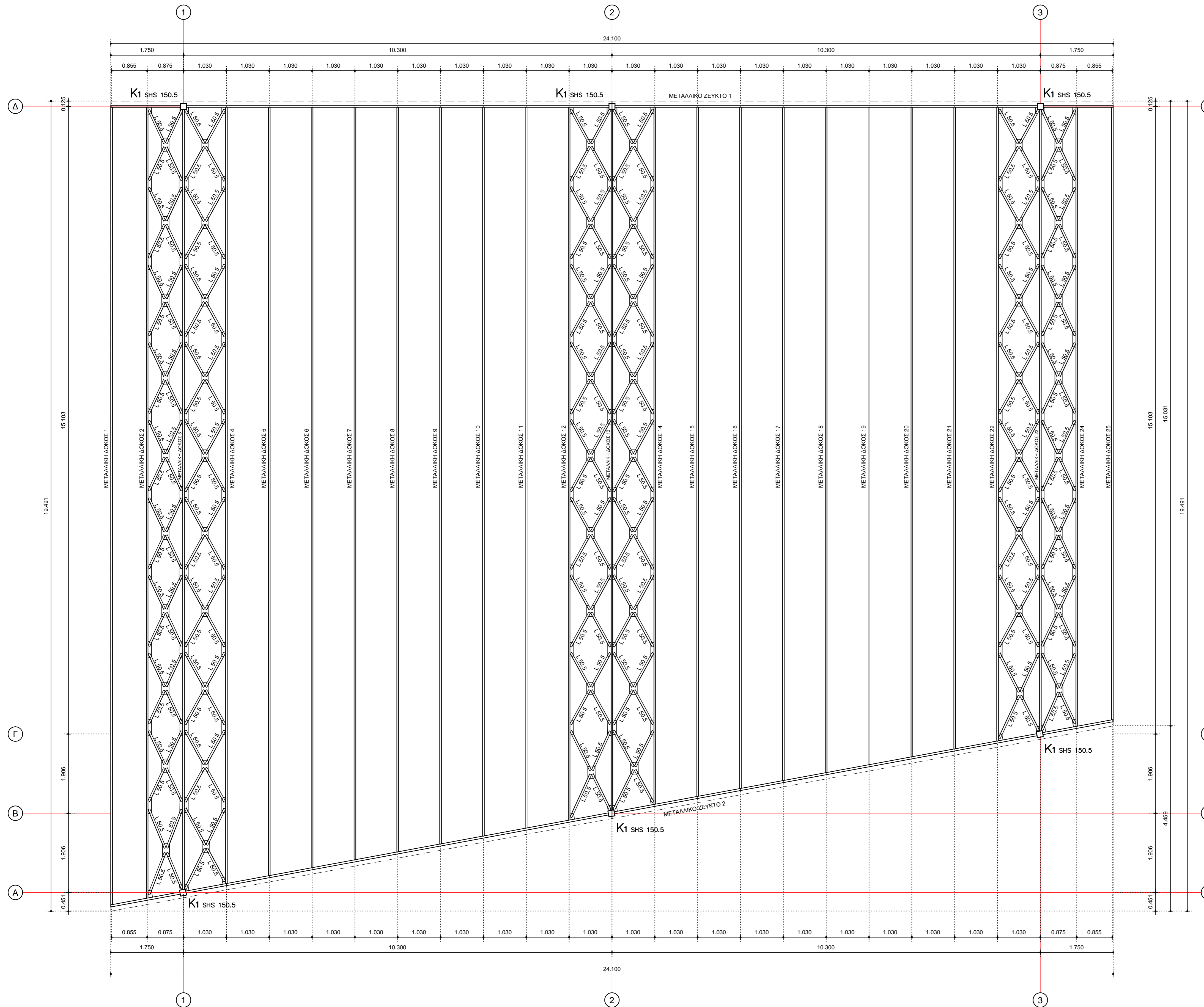
ΚΑΤΟΨΗ ΣΤΕΓΗΣ ΚΛΙΜΑΚΑ 1:50
